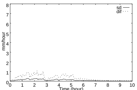
図 8 地表面流：流出高の違い (1000m)
