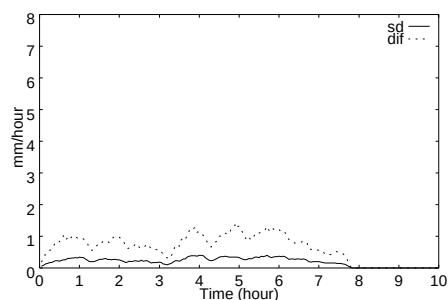
図 5 中間流：流出高の違い (400m)
