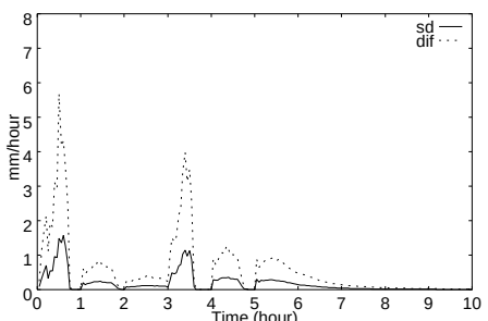
図 7 地表面流：流出高の違い (100m)
