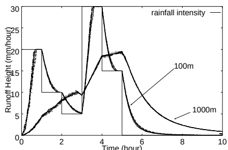
図 6 地表面流：ハイドログラフ
