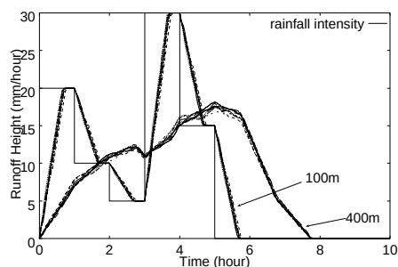
図 3 中間流：ハイドログラフ
