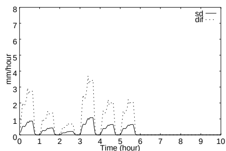
図 4 中間流：流出高の違い (100m)
