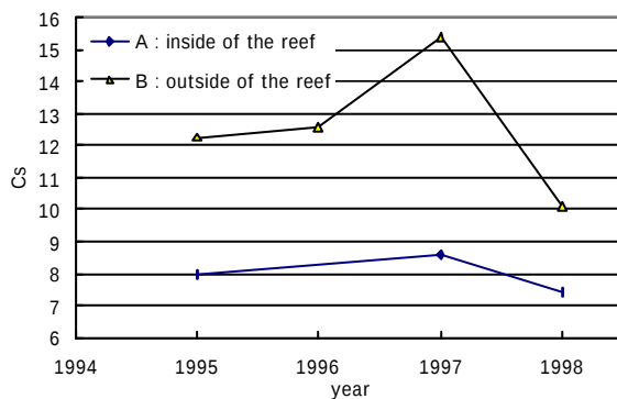
Figure 5 C_s parameter
