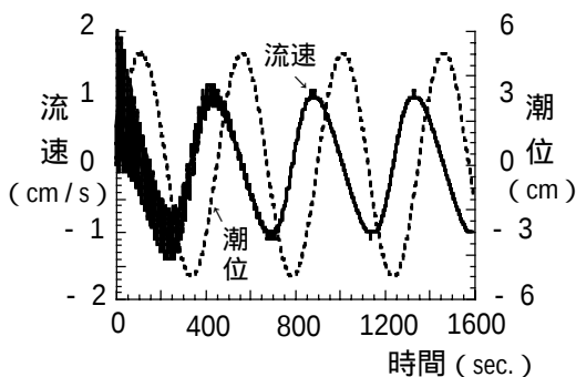
図5 2次元WFDMによる潮位・流速解
