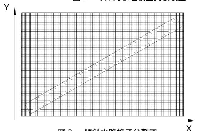
図3 傾斜水路格子分割図
