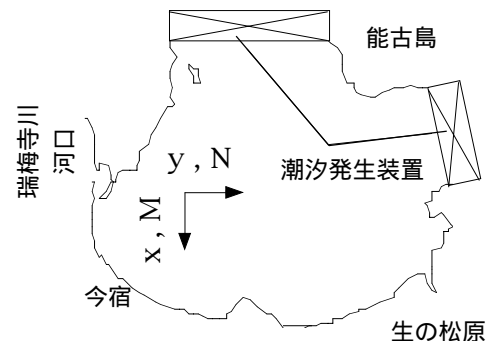
図1 今津湾水理模型実験装置
