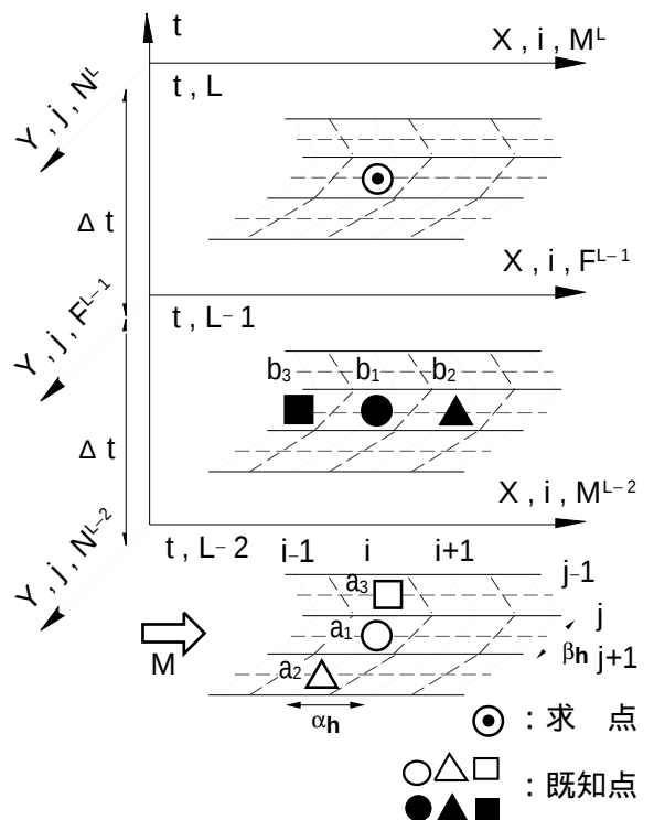
図4 多段階陽形式重み付差分モデル
