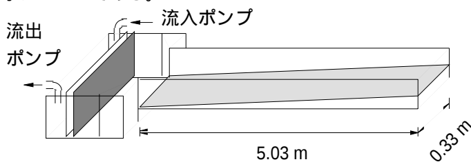
図2 傾斜水路模型実験装置
