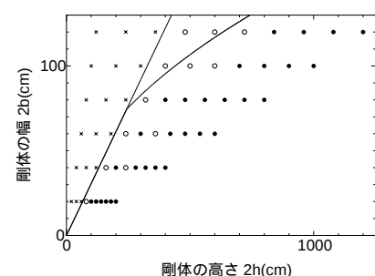
図 7: 地震時の剛体の挙動 図 8: 壁が存在しない場合の挙動 図 9: 壁が存在する場合の挙動
