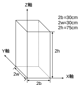
図 1: 3次元剛体のモデル 図 2: 速度振幅一定による転倒条件 図 3: 加速度振幅一定による転倒条件
