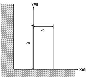
図 4: 2次元剛体のモデル 図 5: 壁が無いときの挙動の例 図 6: 壁の有るときの挙動の例
