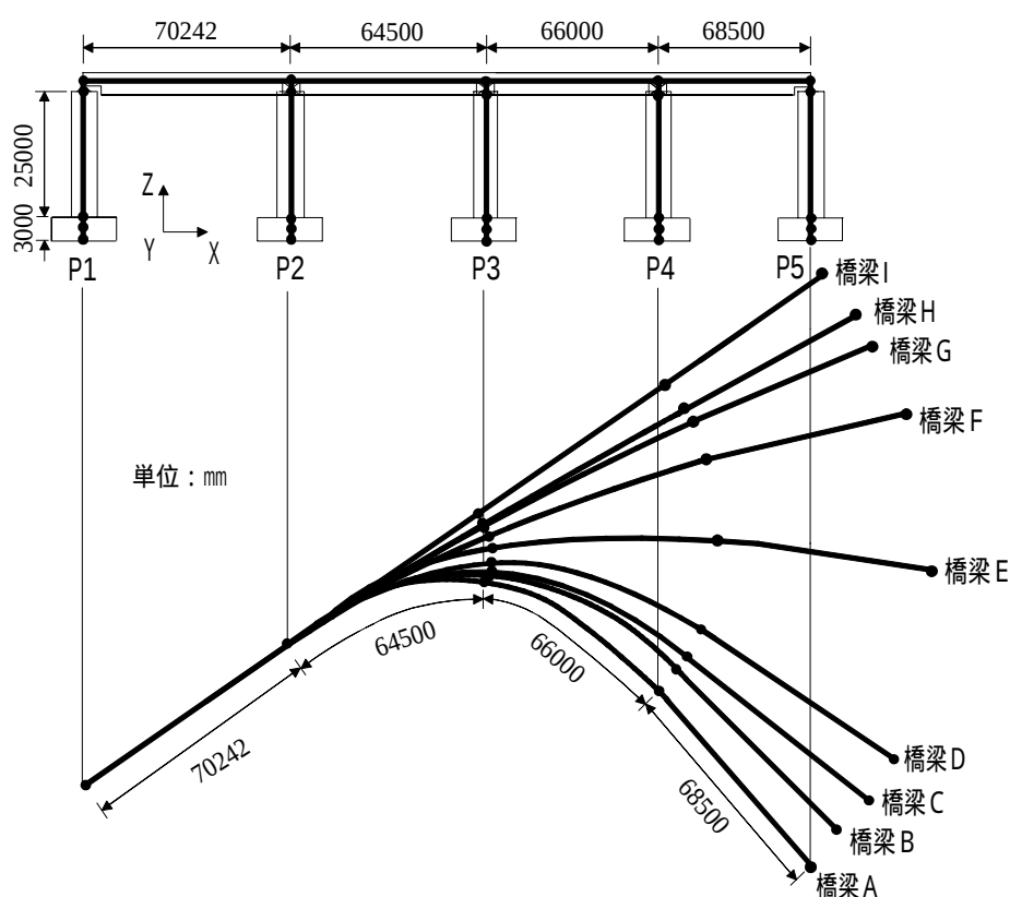
図 1 解析モデル
