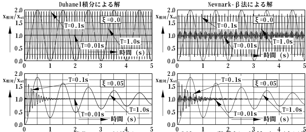
図-2 Duhamel 積分による理論解と Newmark- \beta 法による数値解の比較 (T:固有周期)
