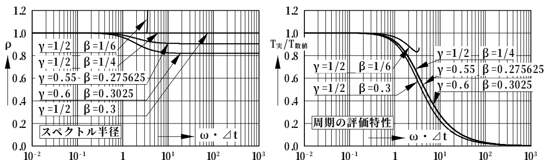
図-1 Newmark-β 法の振幅と周期の評価特性
