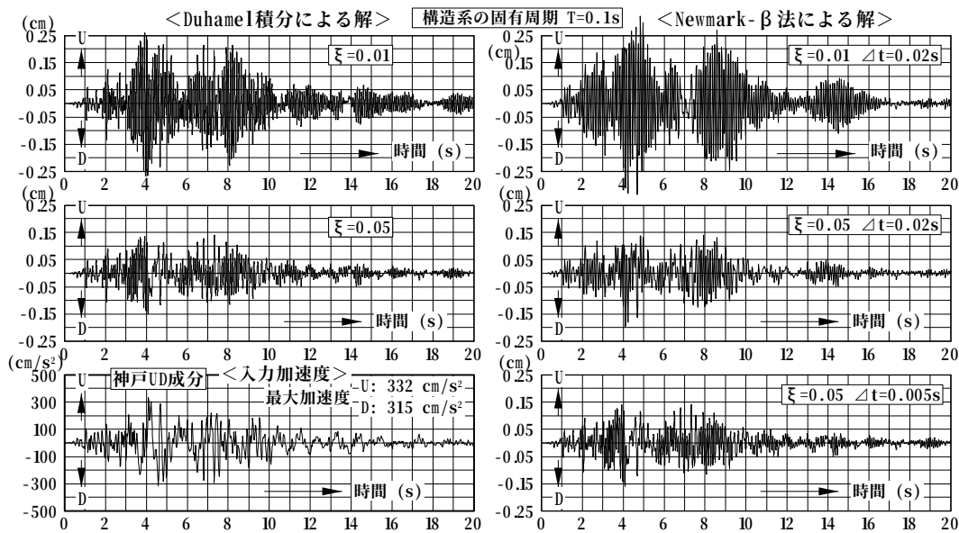
図-3 実地震記録のもとでの応答の Newmark- \beta 法による解と理論解との比較
