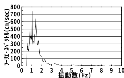
図7 地表面のフーリエ・スペクトル (簡易地盤モデル・第1層～第8層を載せた場合)
