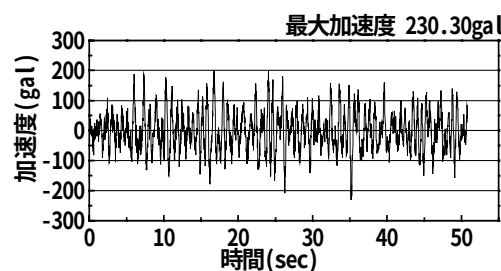
図4 地表面の加速度時刻歴 (1次元重複反射法)
