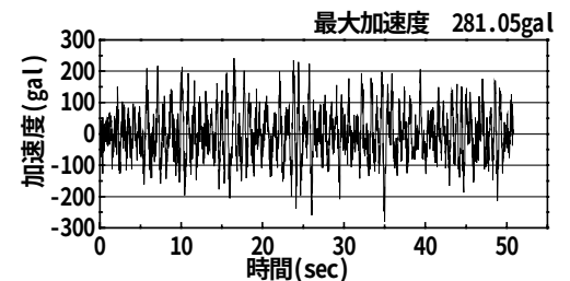
図1 入力地震動の加速度時刻歴
