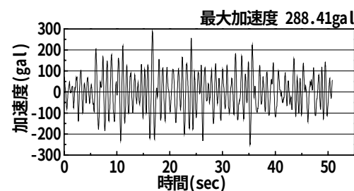
図5 地表面の加速度時刻歴 (簡易地盤モデル・第1層～第8層を載せた場合)
