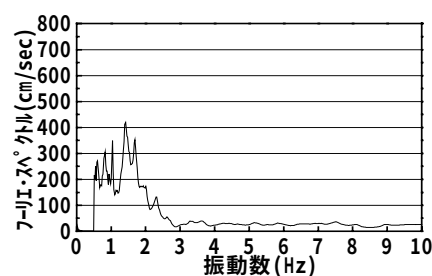
図6 地表面のフーリエ・スペクトル (1次元重複反射法)
