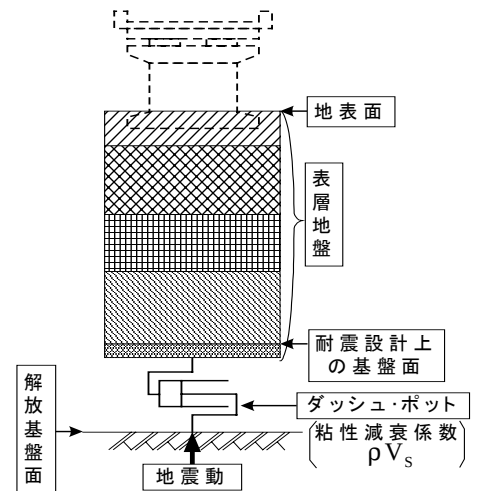
図2 簡易地盤モデル
