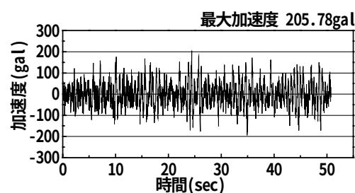
図3 内部基盤面の加速度時刻歴 (1次元重複反射法)
