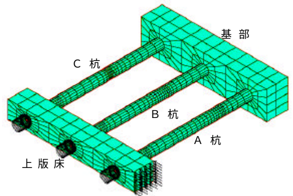
図-4 FEMモデル (2Dモデル)
