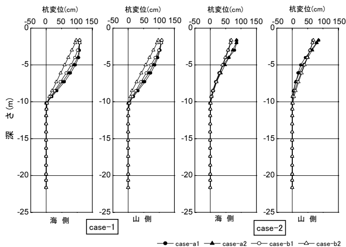
図-5 杭の変位
