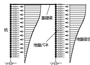
図-2 解析モデル
