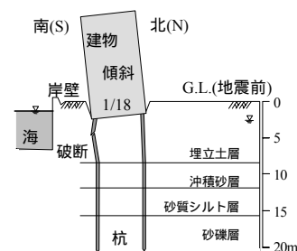
図-1 杭の被害の模式図 (文献1)を参考に描写)
