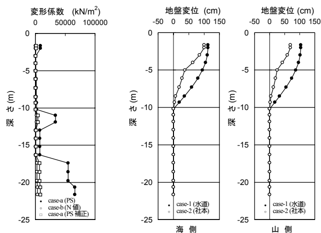
図-3 地盤の変形係数
