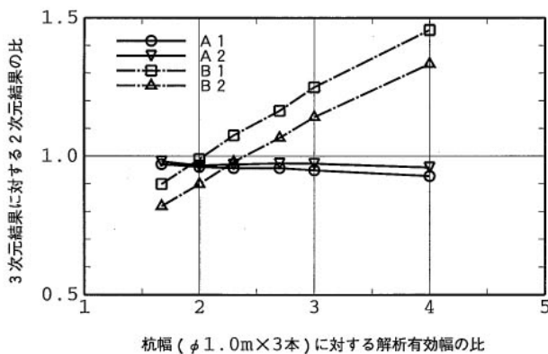
図 - 4 3次元解析結果に対する2次元解析結果の曲げモーメント比と有効幅の関係 (杭径 1.0m)
