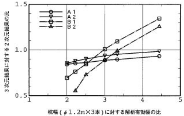
図 - 5 3次元解析結果に対する2次元解析結果の曲げモーメント比と有効幅の関係 (杭径 1.2m)
