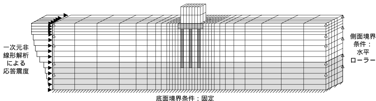
図 - 1 3次元地盤応答震度法の概念図
