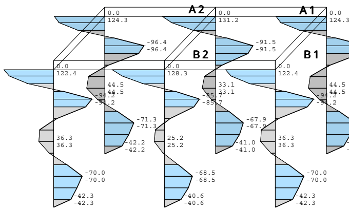
図 - 2 3次元解析結果の曲げモーメント分布
