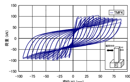
図-4 TMFK 荷重-変位曲線
