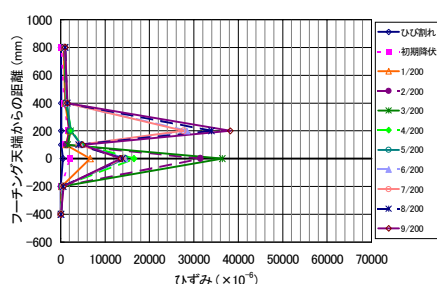
図-5 TC 引張側鉄筋のひずみ分布
