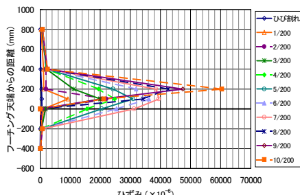
図-6 TMKK 引張側鉄筋のひずみ分布
