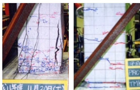
図-8 供試体破壊形状(左: TC 右: PRC Pca)
