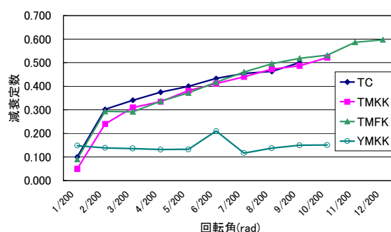
図-10 減衰性能
