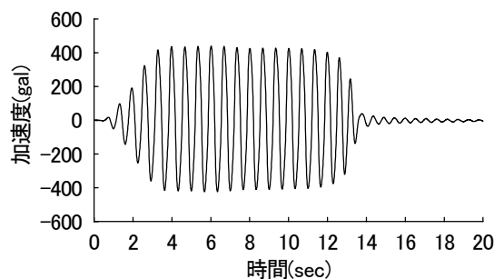
図-2 入力波形
