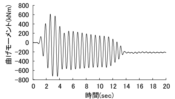
(a) 杭頭部
