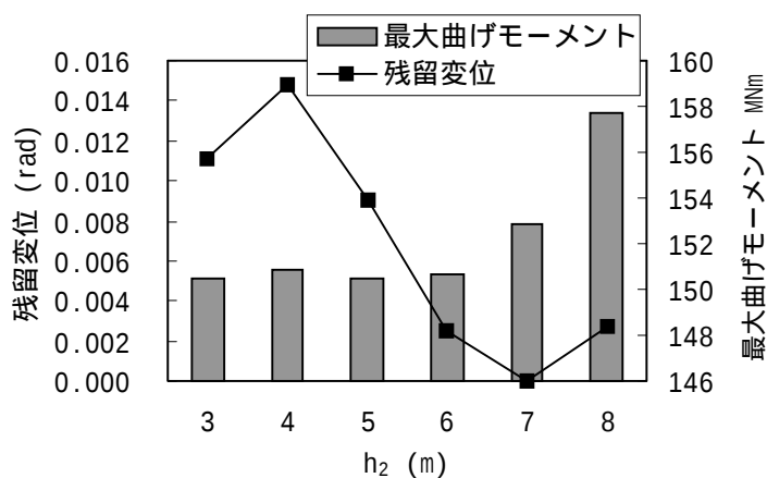
図6 残留変位と最大曲げモーメントの関係
