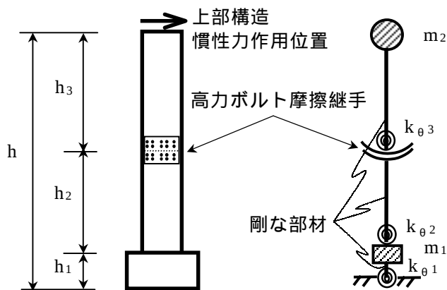
図1 解析対象橋脚
