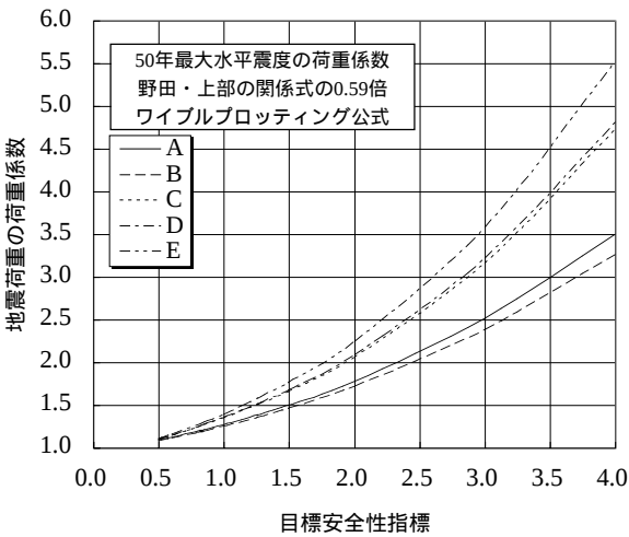
図 - 1 地震荷重の荷重係数と目標安全性指標の関係
