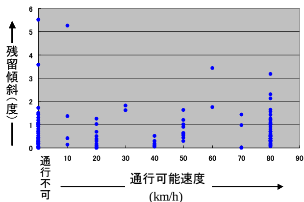
図-4 通行可能速度ごとの橋脚の残留傾斜
