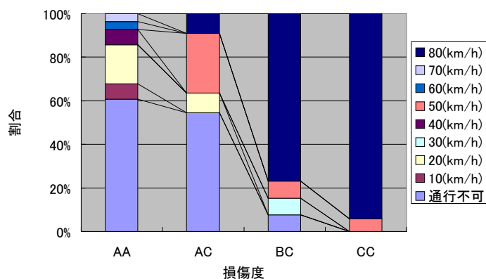
図-6 支承の損傷度ごとの各通行可能速度の割合
