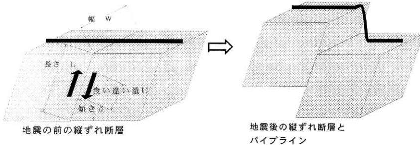
図-1. 地震前後の縦ずれ断層
