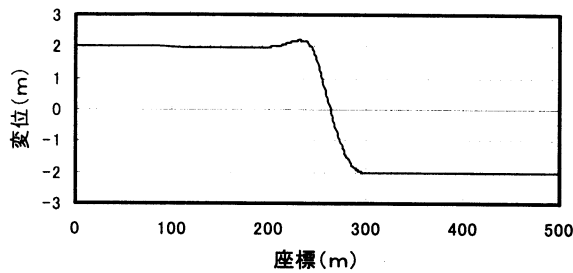
図-3 縦ずれ断層の変位分布図
