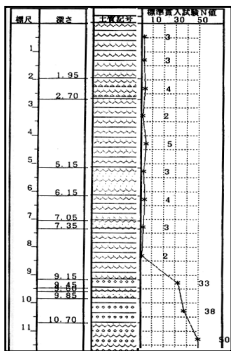
図-5 鮫柱状図
