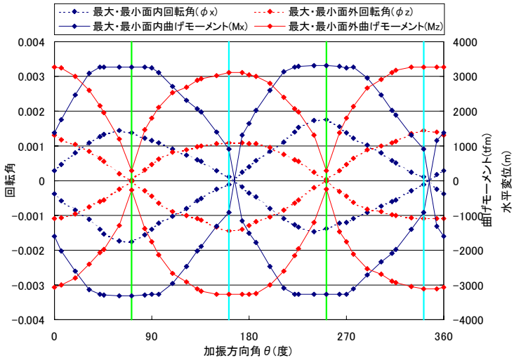
図-5 塑性ヒンジ部の最大・最小曲げモーメントと回転角
