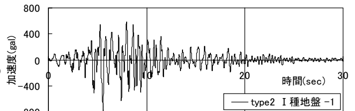
図-2 入力加速度波形
