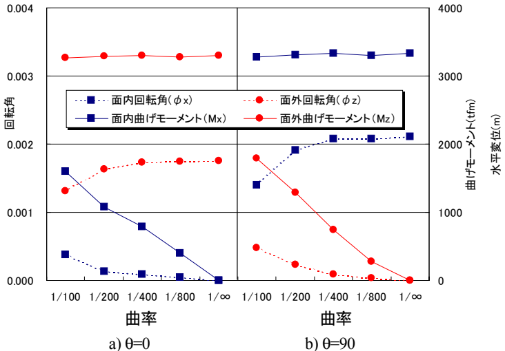
図-7 塑性ヒンジ部の最大曲げモーメントと回転角
