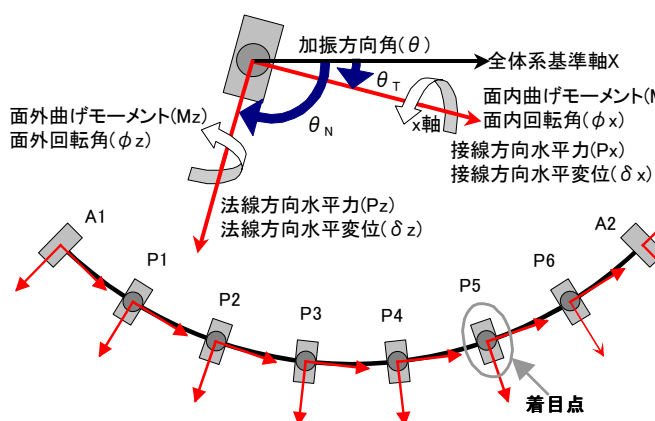
図-3 地震動の加振方向と座標の定義
