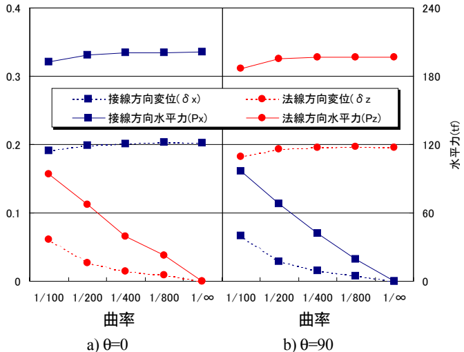
図-8 免震支承部の最大水平力と水平変位
