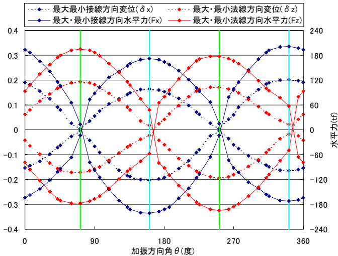
図-6 免震支承部の最大・最小水平力と水平変位
