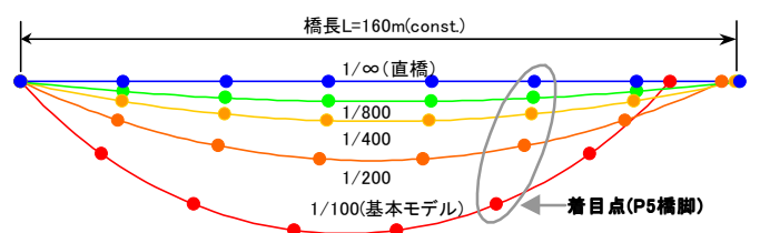
図-4 曲率を変化させた解析モデル
