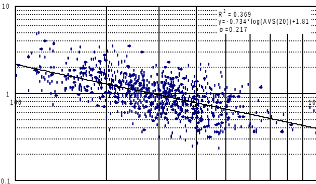
図3 PGV 増幅度と地盤増幅度の関係
