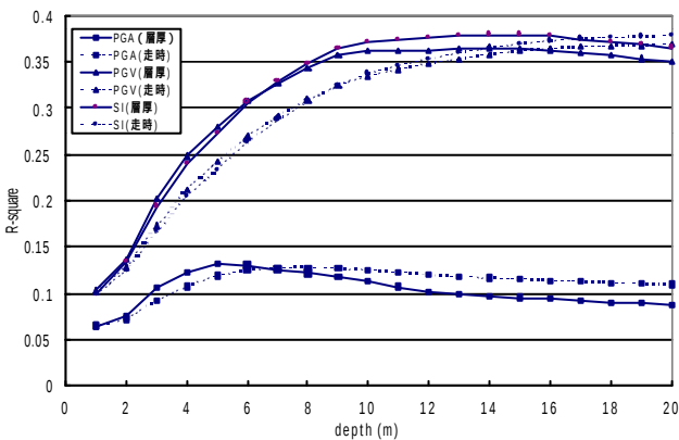
図2 AVS と地盤増幅度の相関の深さ方向の変化
