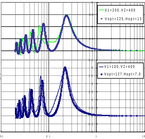
図1 3 層系と等価な 2 層系の伝達関数の比較
