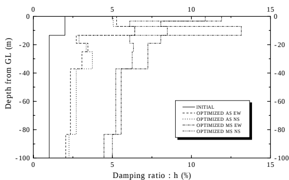
図5 余震、本震同定解析で求まった減衰比の比較
