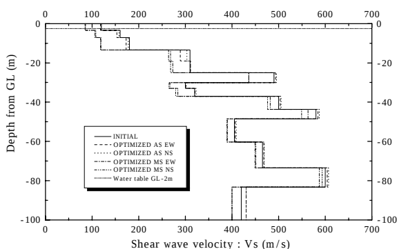
図4 余震、本震同定解析で求まった S 波速度の比較
