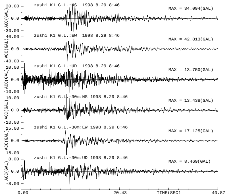
図2 地震観測データ(8/29/98)
