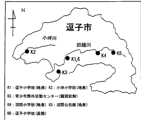
図1 強震アレー観測点
