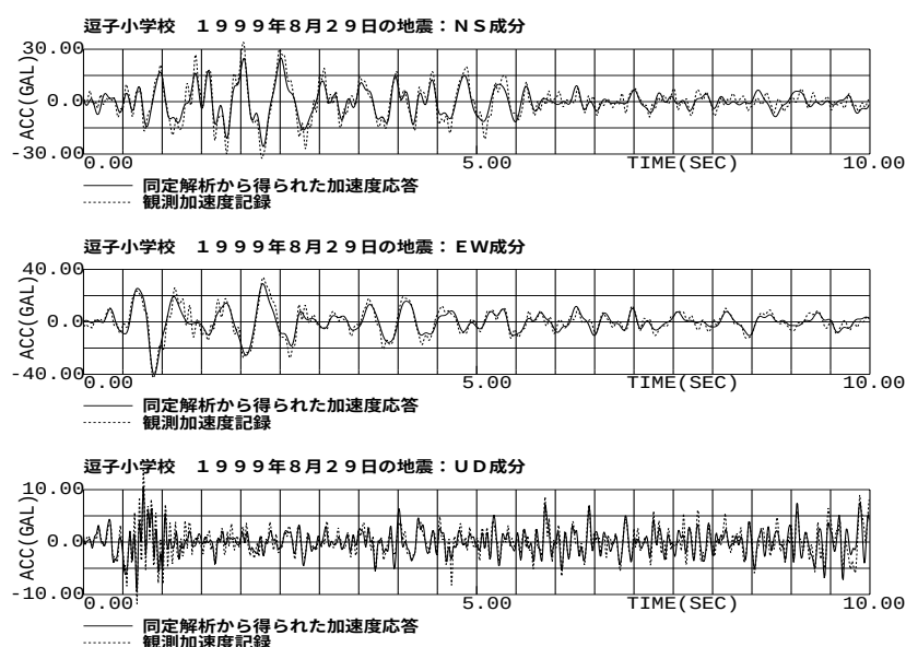
図4 加速度応答波形の観測値と同定解析値の比較
