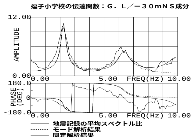
図3 伝達関数の観測値と解析値の比較
