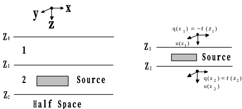
図－1 震源断層を含む成層地盤と記号
