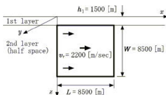
図－2 震源断層—地盤モデル
