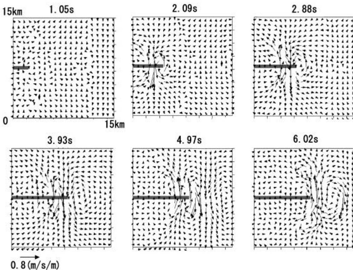
図－3 時間毎の地表面水平速度の空間分布
