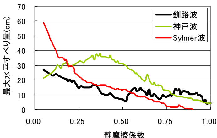
図1 設置面での静摩擦係数と最大水平すべり量
