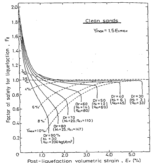
図-1 液状化危険度と体積ひずみの関係 3)
