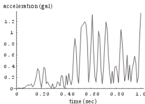
図2.(a) 特定方向成分のノルム
