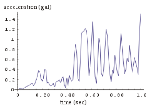
図2.(b) 3方向合成のノルム
