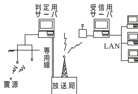
図1. 即時警報システムの概要
