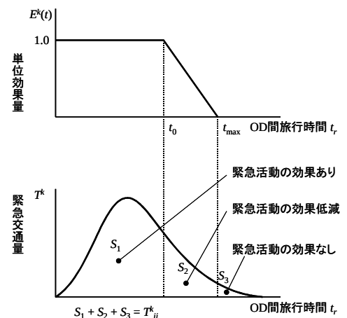
図1 道路ネットワーク耐震性の考え方
