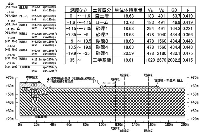
図－１ 二次元等価線形解析モデル
