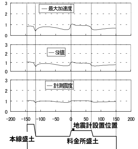
図－３ 二次元等価線形解析結果
