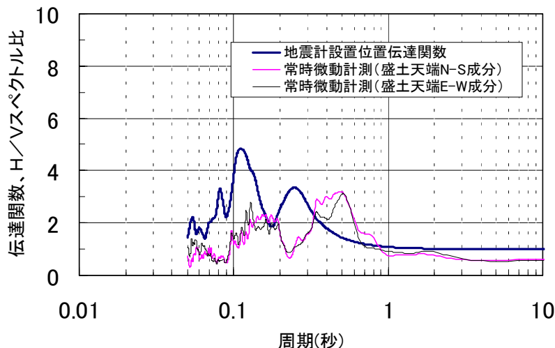
図－２ 伝達関数と常時微動H/Vスペクトルの比較
