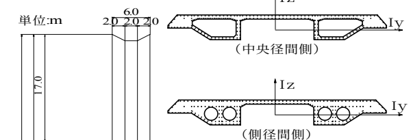
図-3 主桁断面
