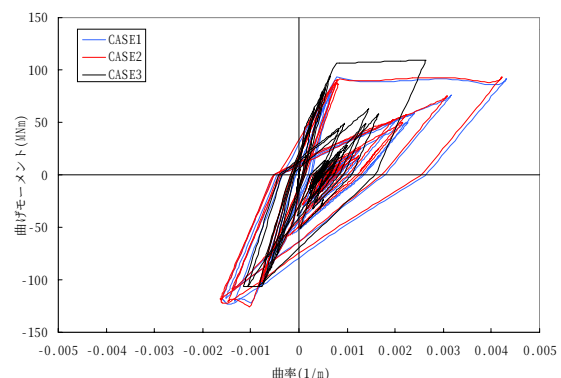
図-8 橋脚基部のM- \phi 履歴曲線
