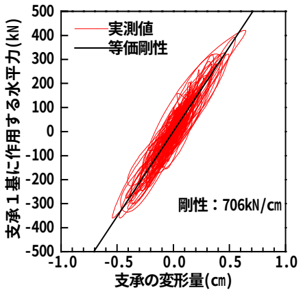
図-4 地震記録から求めたゴム支承の荷重-変形図、等価剛性
