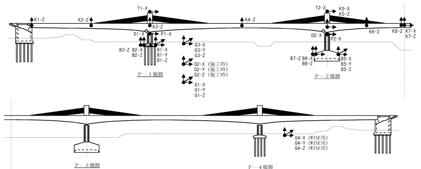
図-1 土狩大橋の地震計設置位置
