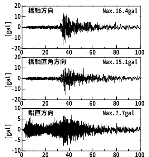
図-2 地盤の加速度記録 (P4 橋脚近傍地盤)
