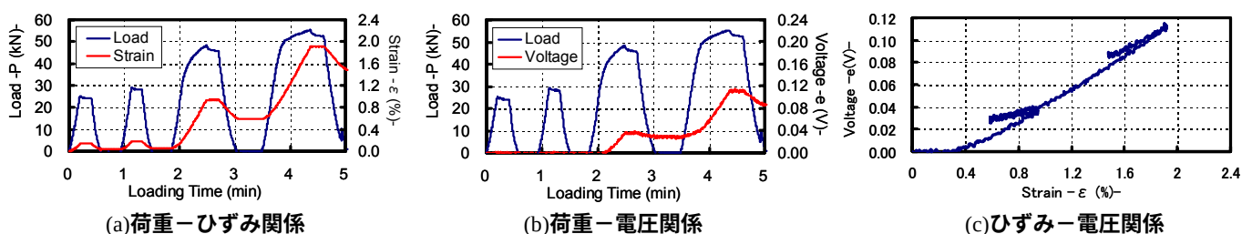
図-5 TRIP 鋼鉄筋の荷重-ひずみ-出力電圧の関係
