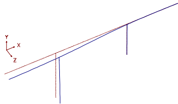
図-5 ラーメン橋変形図（面外方向）
