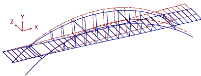
図-9 アーチ橋変形図（面外方向）
