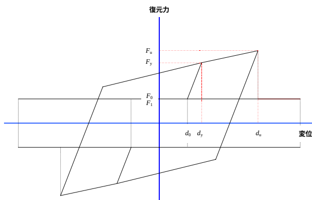
(a) 固定支承, および可動支承の橋軸直角方向モデル
