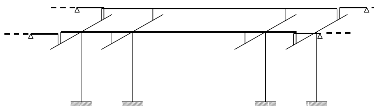
図 4 解析モデル
