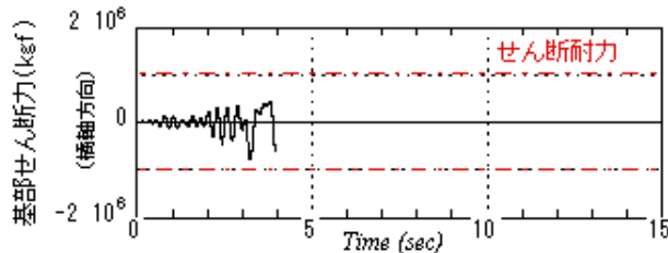
(b) 支承の破壊を考慮した場合の P270 橋脚基部における橋軸方向のせん断力
