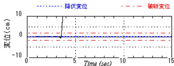
(c) 支承の破壊を考慮した場合の P270 橋脚上ピン支承の橋軸直角方向変位
