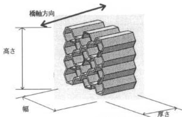
図－3 ハニカム型緩衝装置
