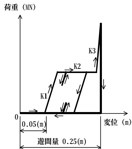
図－4 緩衝装置の履歴モデル
