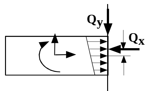
図3 全面で衝突する場合
