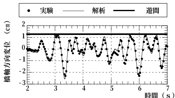
図5 1次元の衝突
