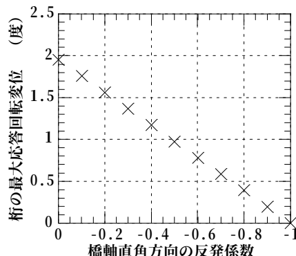
図8 橋軸直角方向の反発係数と回転変位の関係
