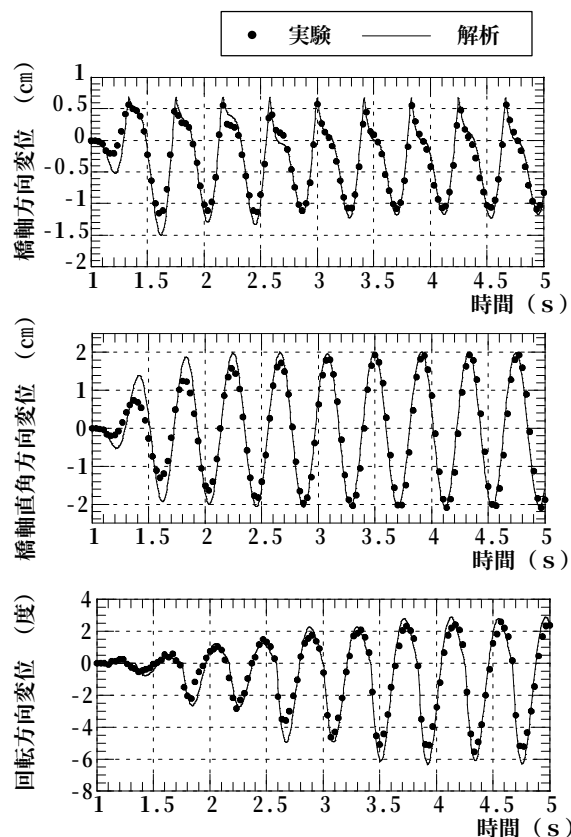
図6 2次元的な衝突
