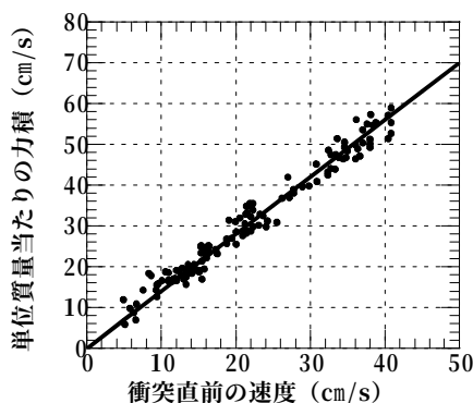
図4 橋軸方向の力積（角度なし）
