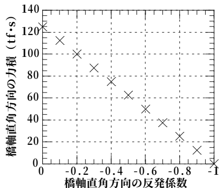
図7 橋軸方向の反発係数と力積の関係
