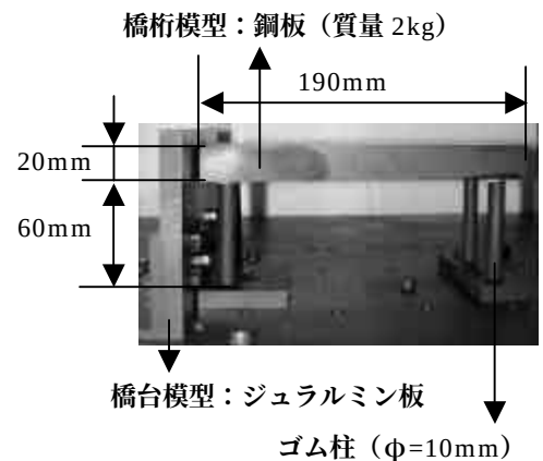
図1 実験模型
