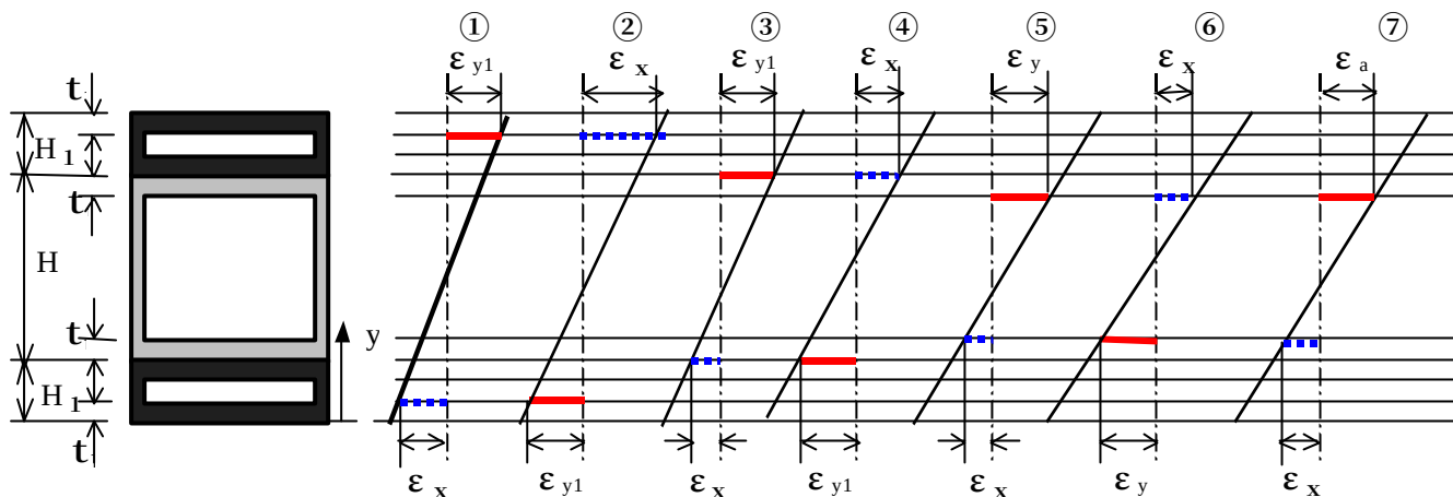
図－４ 断面平面保持の法則による各ひずみ計算過程
