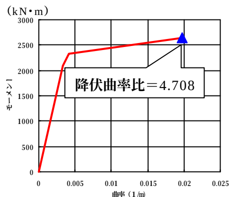
図－５ 橋脚断面の骨格曲線と最大応答値
