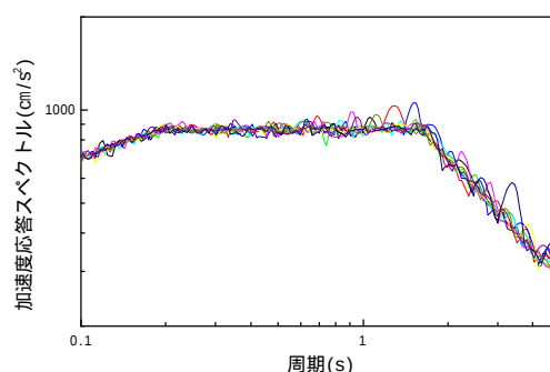
図-2 模擬地震波の加速度応答スペクトル
