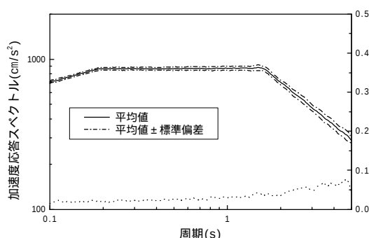
図-3 加速度応答スペクトルの統計値
