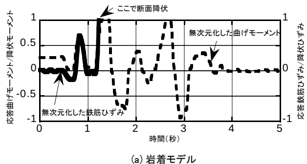
図-5 降伏した要素での実験／解析結果の比較(左側壁下端)
