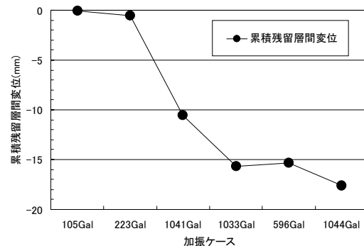
図-6 累計残留層間変位
