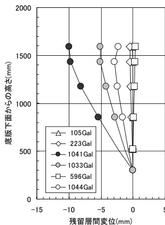
図-5 試験体位置での残留層間変位分布
