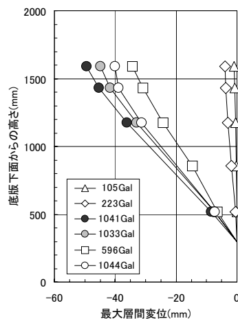
図-4 試験体位置での最大層間変位分布
