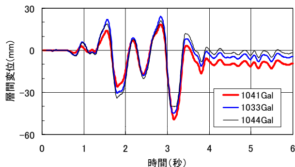
図-2 層間変位の時刻歴波形
