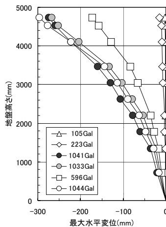
図-7 地盤の最大水平変位
