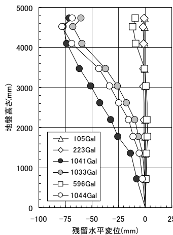
図-8 地盤の残留水平変位
