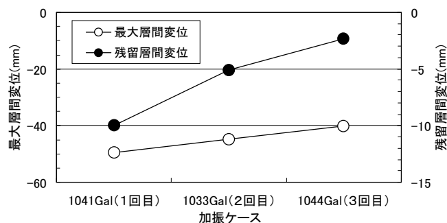
図-3 最大層間変位および残留層間変位
