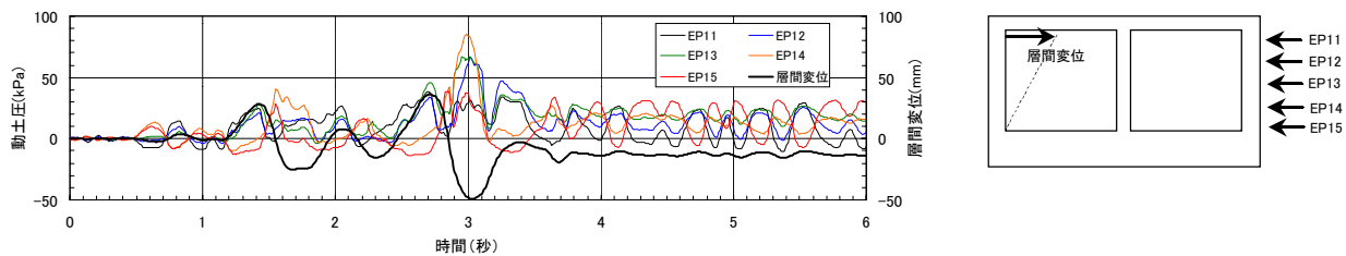
図-3 試験体の層間変位と側壁（右側）に作用する動土圧の時刻歴波形
