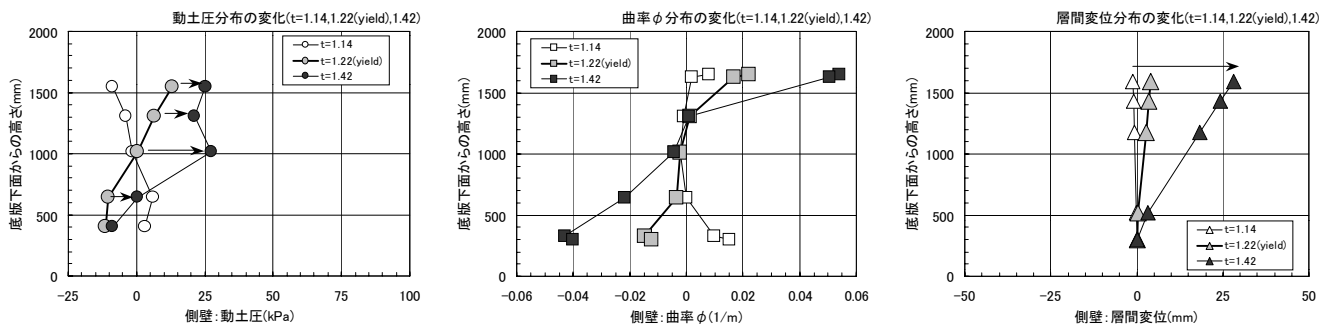
図-5 側壁（右側）に作用する動土圧、曲率および層間変位の分布の変化（降伏変位時刻）
