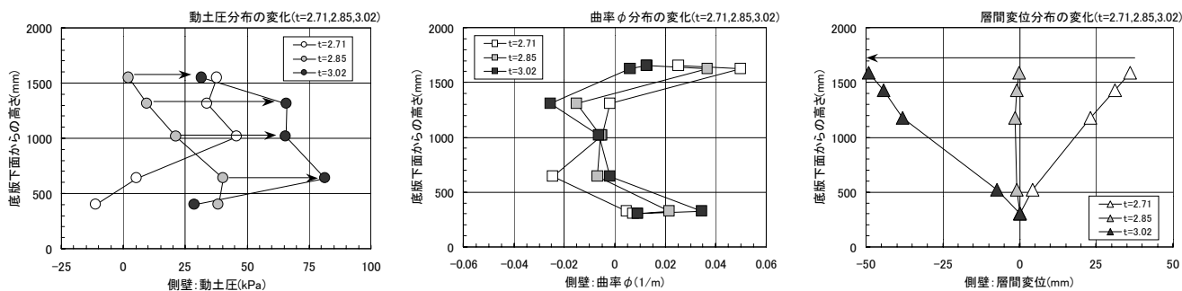
図-6 側壁（右側）に作用する動土圧、曲率および層間変位の分布の変化（最大変位時刻）
