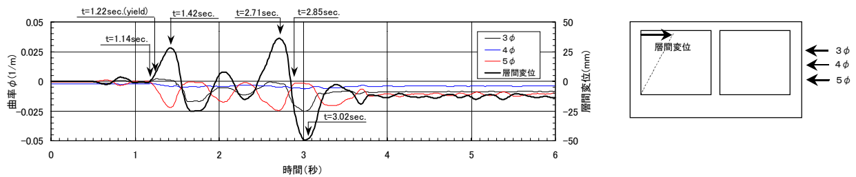
図-4 試験体の層間変位と側壁（右側）の曲率の時刻歴波形
