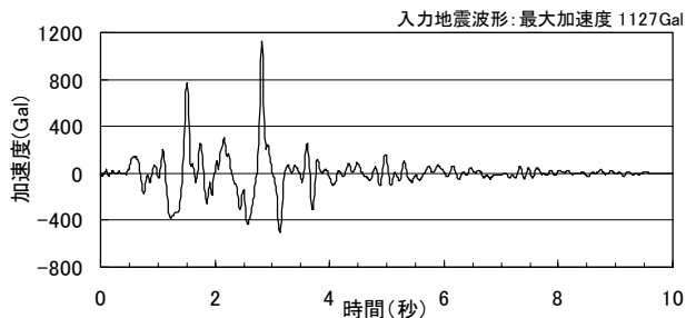
図-2 振動台入力加速度波形
