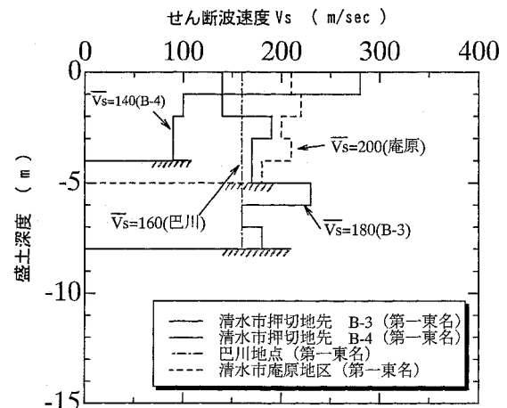
図-2 JH既設盛土の原位置調査結果（P S 検層）
