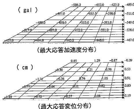
図-3 三次元応答解析結果
