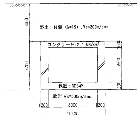
図-4 検討対象ボックスカルバート構造断面
