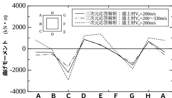
図-5 断面力比較図（曲げモーメント）
