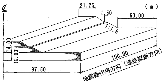
図-1 三次元応答解析モデル
