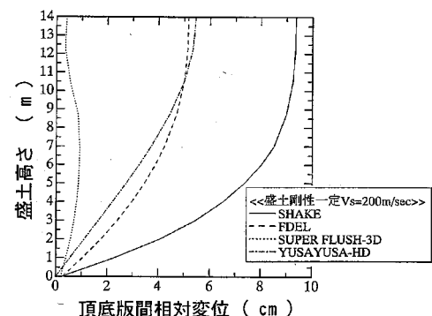
図-6 頂底板間相対変位の比較図
