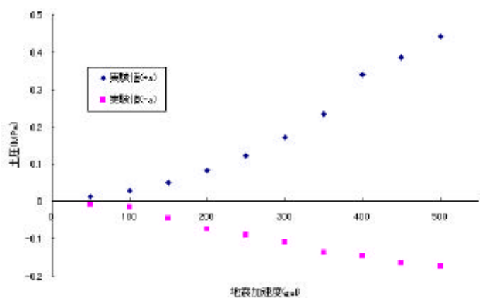
図3 下部動土圧
