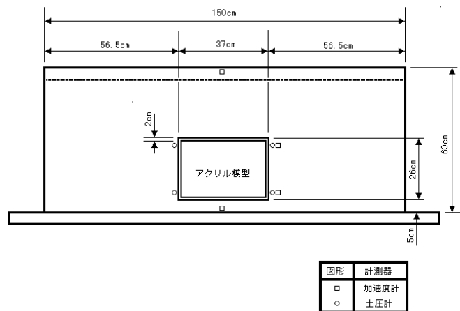
図1 土層図
