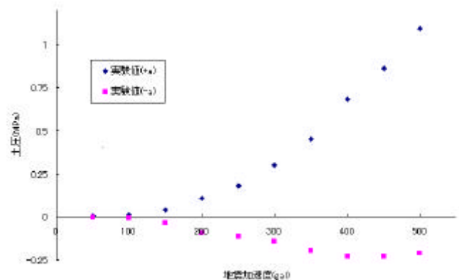
図2 上部動土圧
