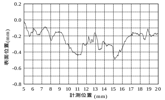
図-3 表面凹凸形状
