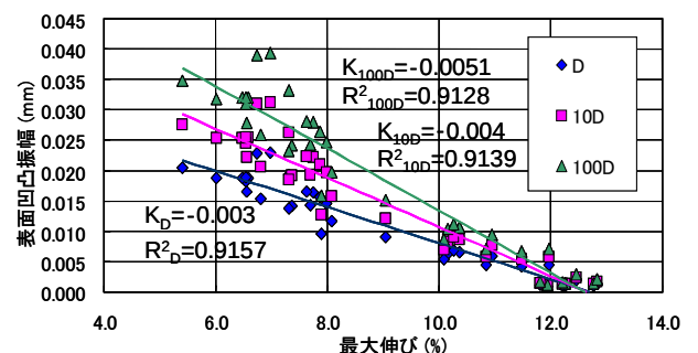
図-6 表面凹凸振幅と最大伸びの関係
