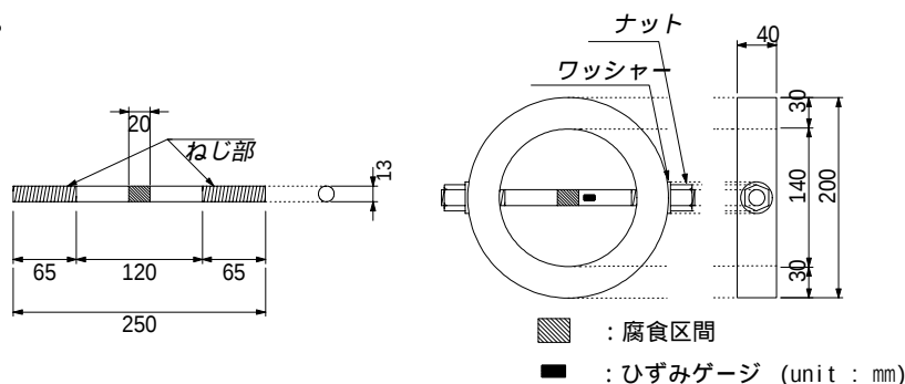
図 - 1 供試体概要
