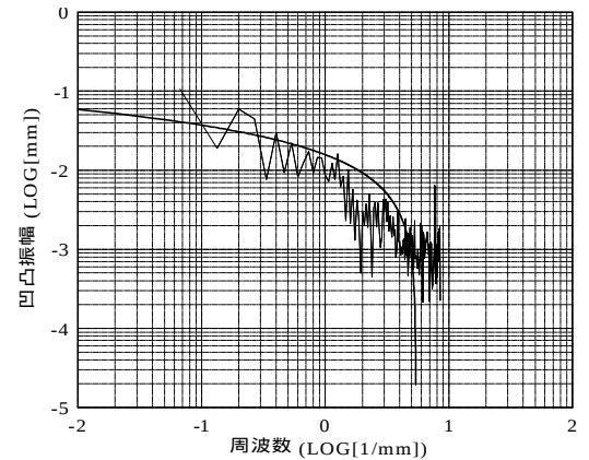
図-4 表面凹凸周波数特性
