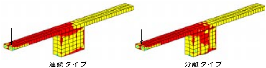
図4 静的解析時の隅角部および床版の主応力の流れ
