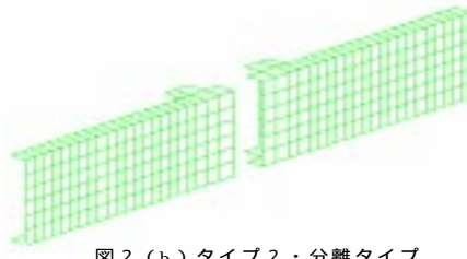
図2(b) タイプ2・分離タイプ
