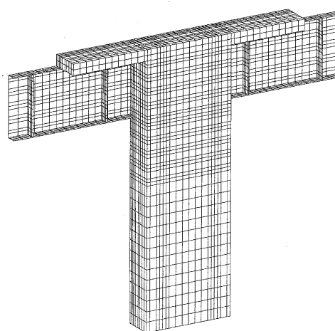
図-3 立体有限要素解析モデル図
