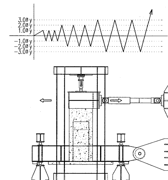
図-2 実験要領図
