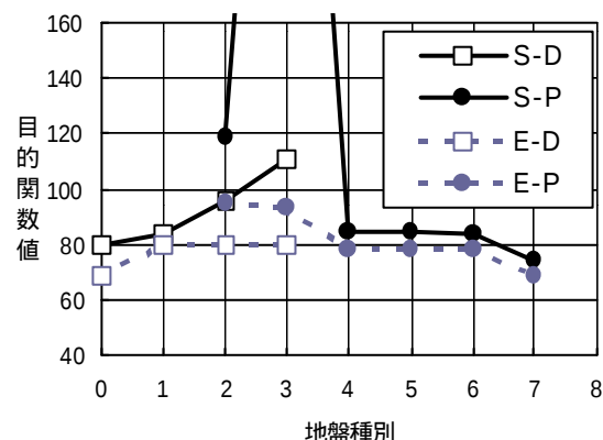
図 - 3 地盤種別による最適解の目的関数値
