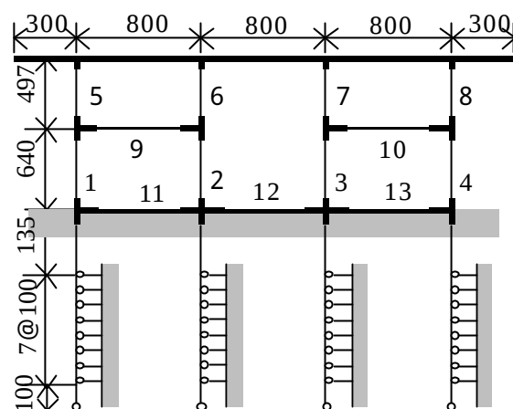
図 - 2 杭基礎構造 RC ラーメン高架橋 (cm)
