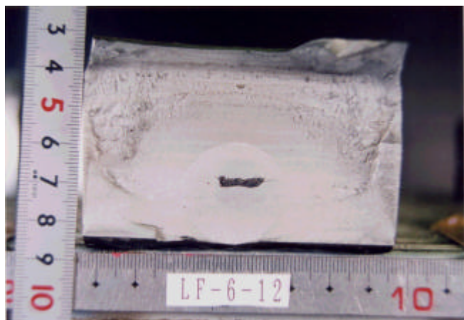
写真-1 破断面(LF試験体)
