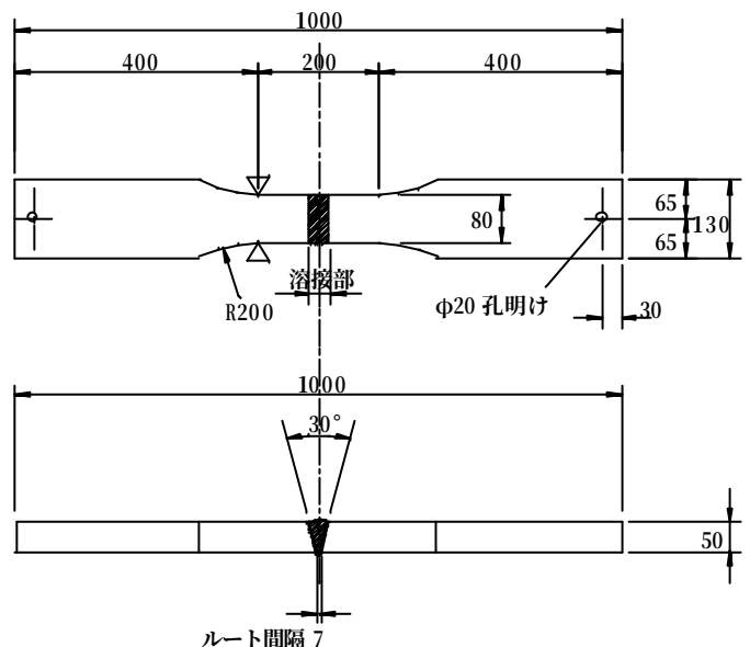
図-1 試験体形状 (50mm試験体)
