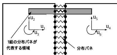
図1 AEMの要素と分布バネ
