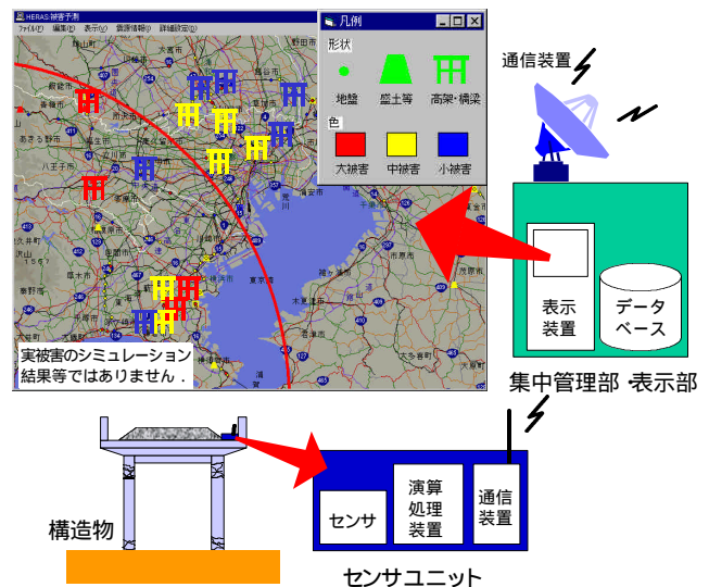
図4 地震被害把握システムの概要
