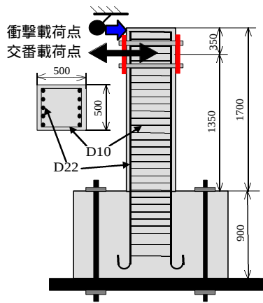
図2 供試体形状及び配筋
