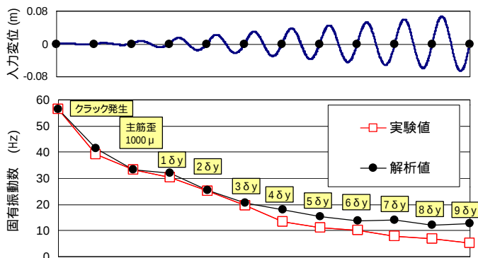
図3 入力波(上図)と損傷による固有振動数変化(下図)
