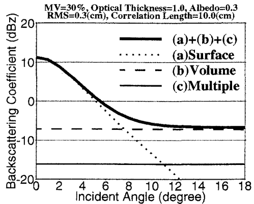
図3 植生のある面からの散乱の計算例
