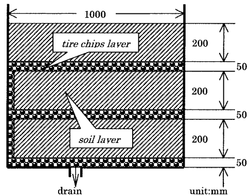
図 1 実験地盤の側面図(ケースB)
