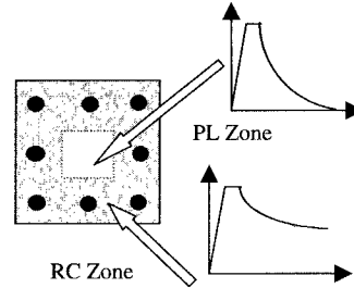
Fig. 3. RC zoning (An et al, 1996)
